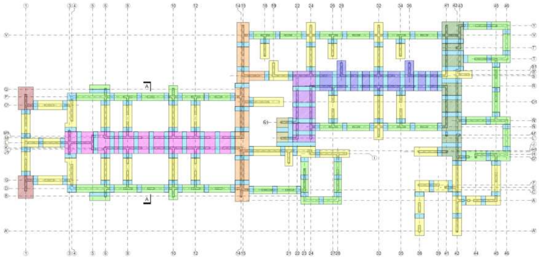
PLANTA GENERAL DE FUNDACIONES 892/1102
